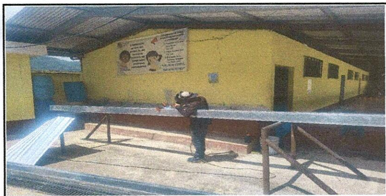
Foto 5: Se efectuaron las labores de soldadura en las vigas principales y costaneras metálicas que conforman la estructura.
