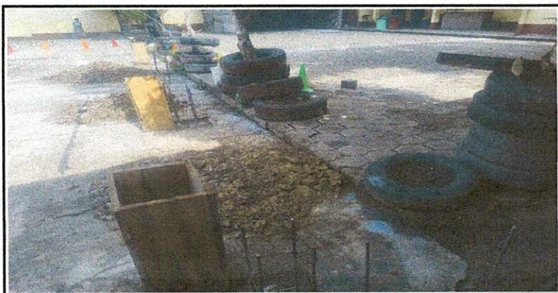
Foto 3: Se realizó la fundición de columnas estructurales que soportaran el peso del entechado a realizar.
